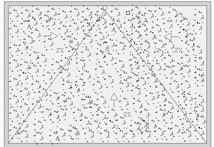
COBERTA
